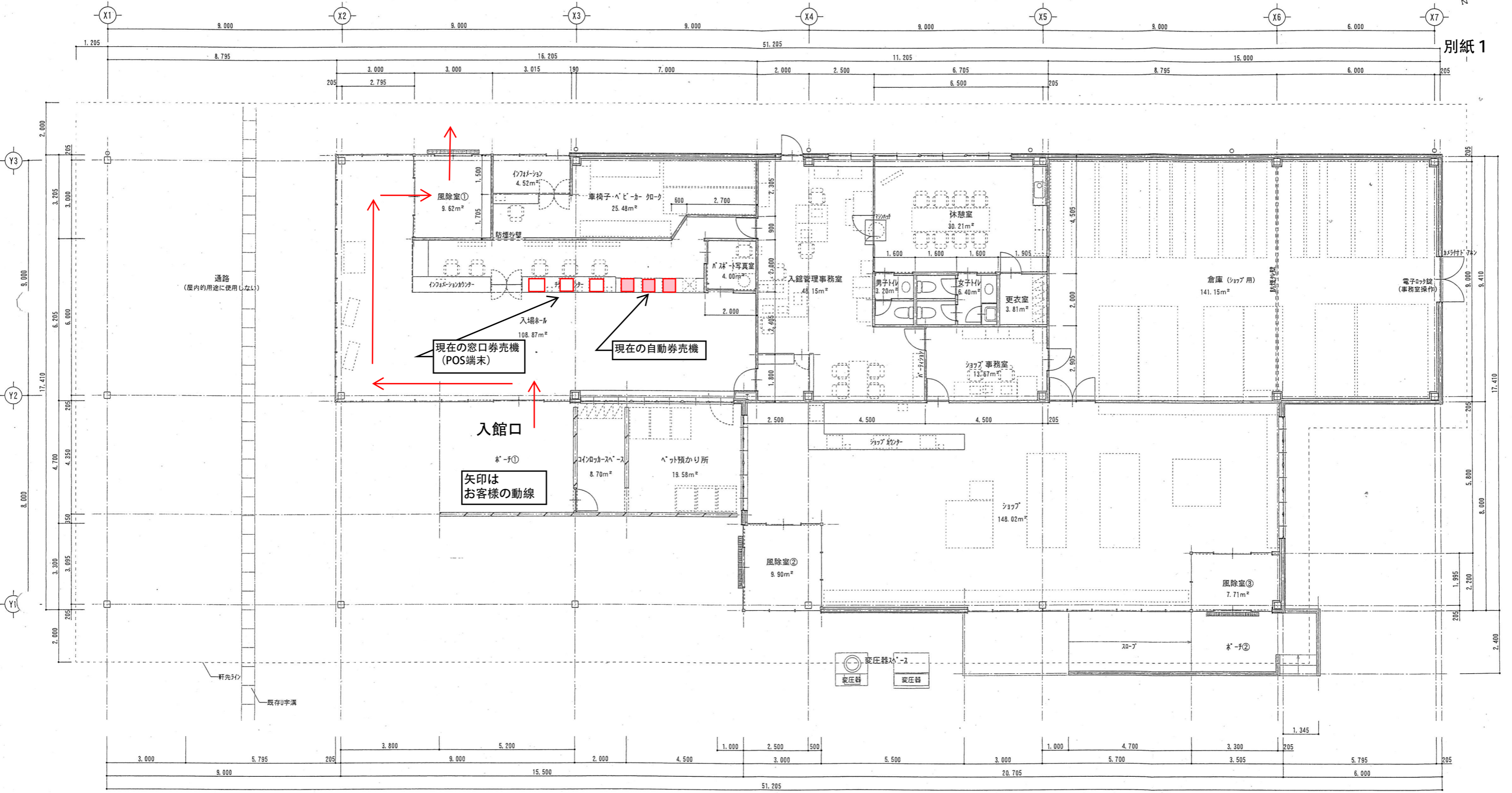
平面図 S=1:100
